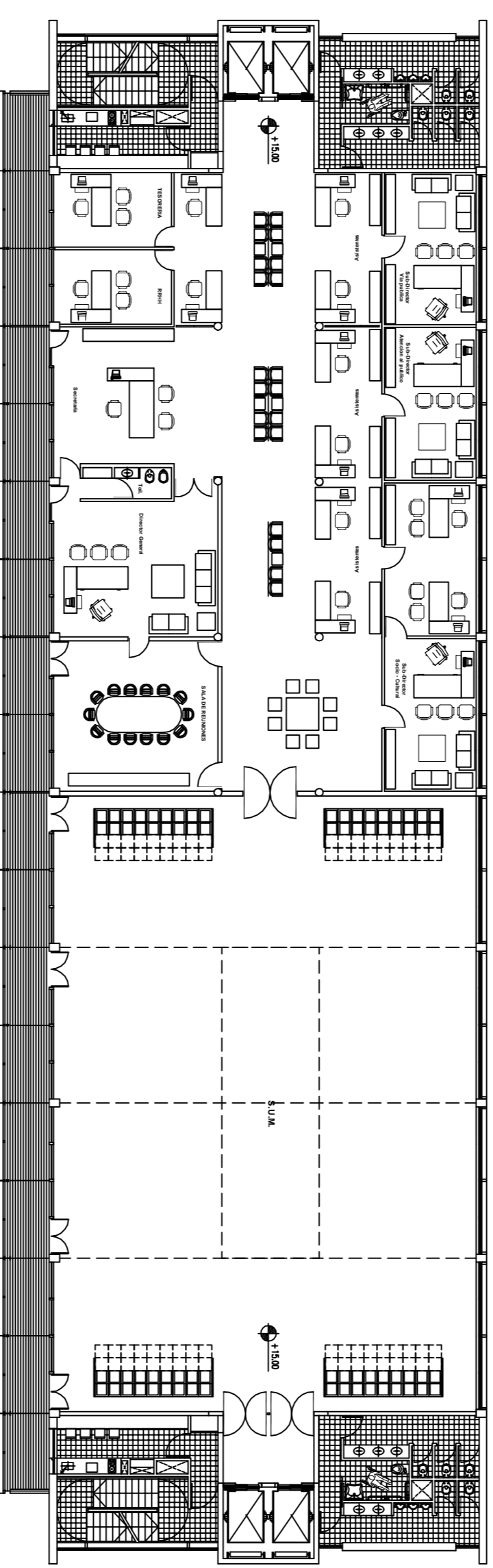
PLANTA 3º PISO
